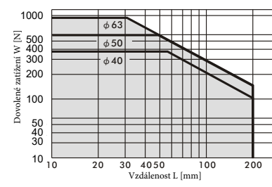
Zdvih 75 až 100 mm
