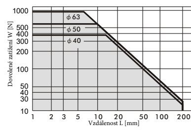
Zdvih 25 až 50 mm
