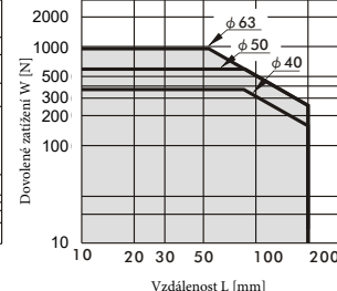
Zdvih 75 až 100 mm
