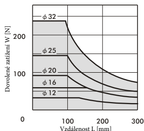
Zdvih 75 až 200 mm
