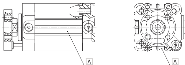
A Snímač polohy musí být umístěn v drážce nejbližší teleskopické tyči
