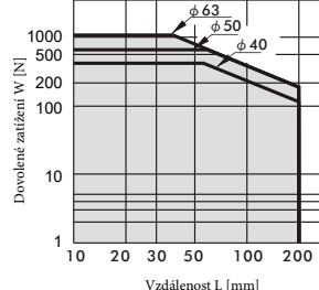
Zdvih 25 až 50 mm
