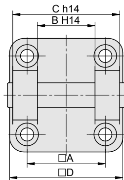
Oko válce přímé (strana 4-8)
