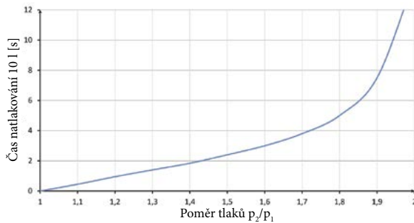
Charakteristika plnění
